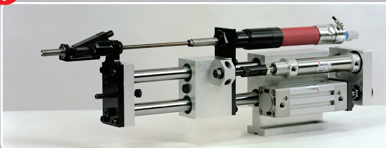
Esempio di avvitatore autoalimentato con applicazione di portainseriti ed inserto filettati (per gentile concessione di MTA TECH S.r.l.) Example of self-powered screwdriver with application of bit holder and threaded insert (by kind permission of MTA TECH S.r.l.)
